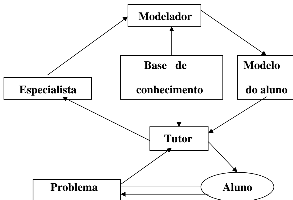
Figura 6 – Arquitectura de um ITS segundo Clancey
